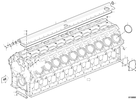
CRANKCASE X00030264
